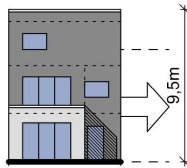
achtergevel
